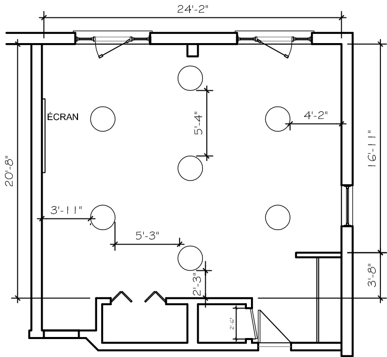
Plan Salle Réunion 138 Aménagement COAKTAIL échelle: 1/4" = 1'-0" environ 28 personnes
