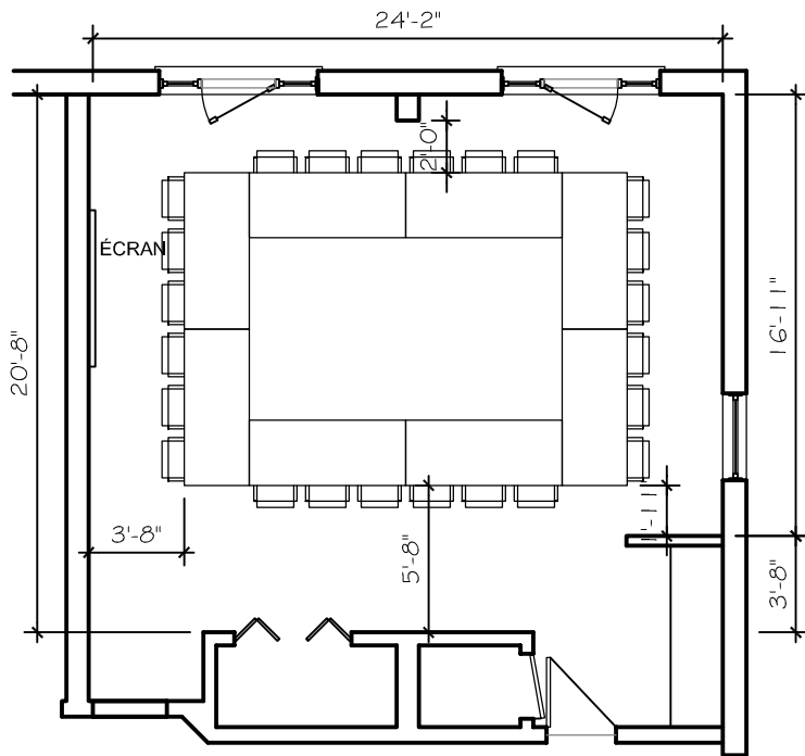
Plan Salle Réunion 138 Aménagement COAKTAIL échelle: 1/4" = 1'-0" environ 28 personnes
