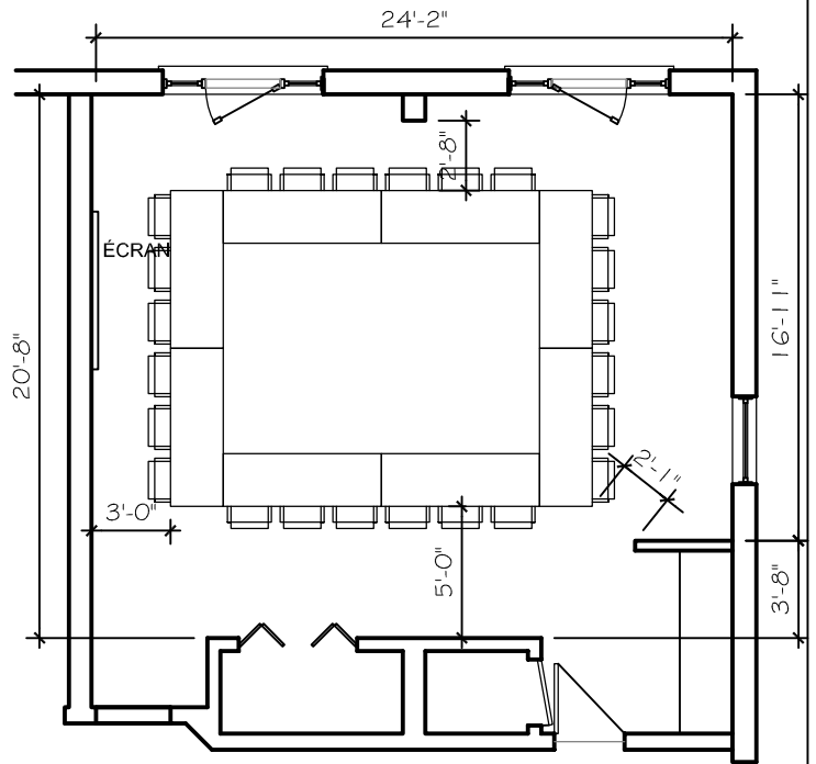
Plan Salle Réunion 138 Aménagement CARRÉ (avec tables de 24" x 72") échelle: 1/4" = 1'-0" 24 personnes
